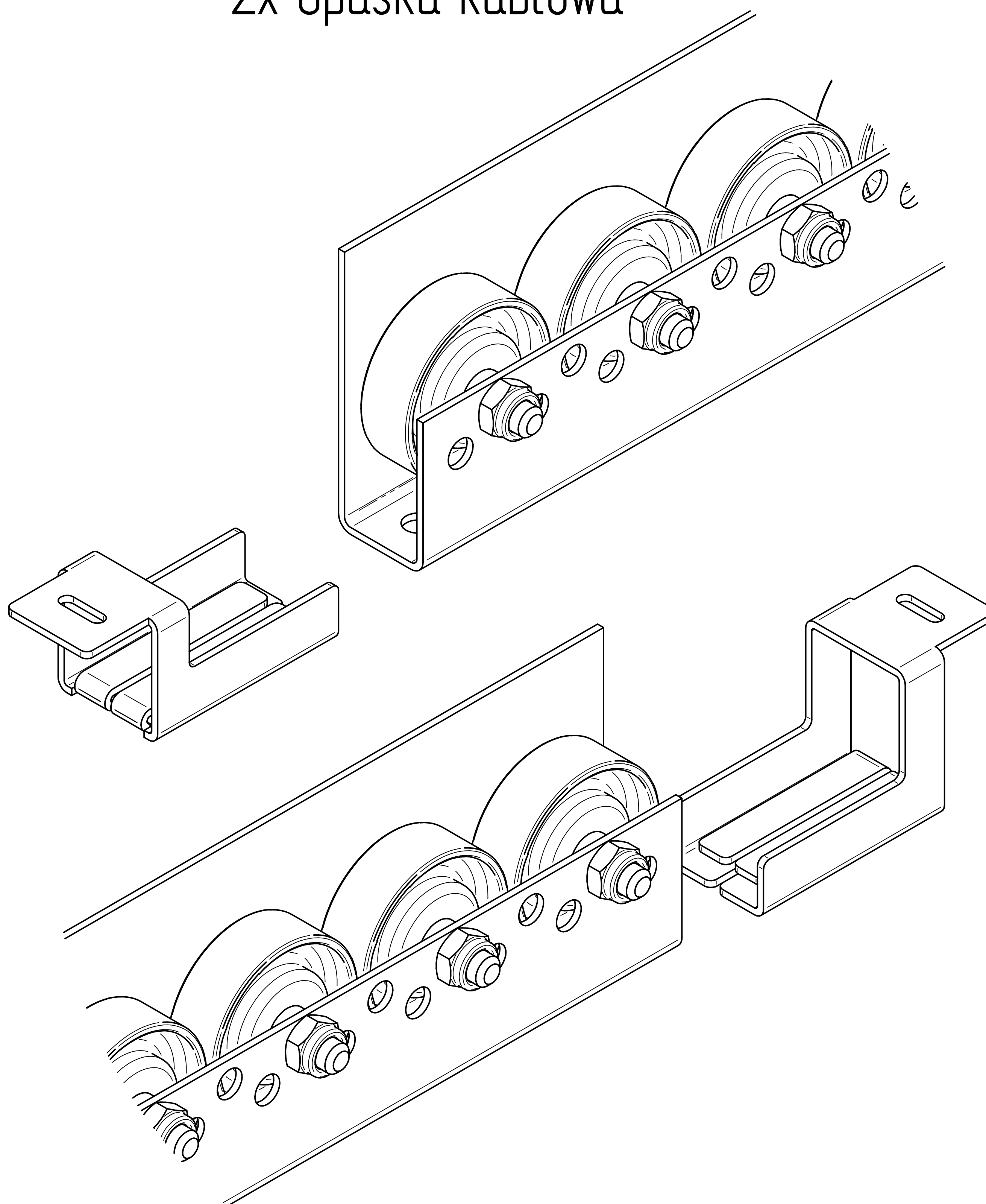
2x Opaska kablowa
